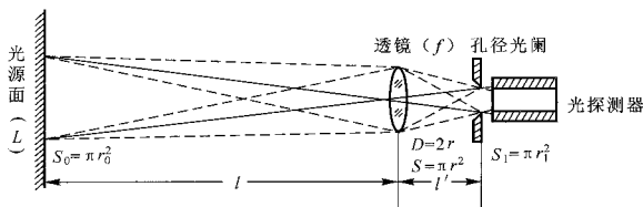
图 1 成像式亮度计结构原理
